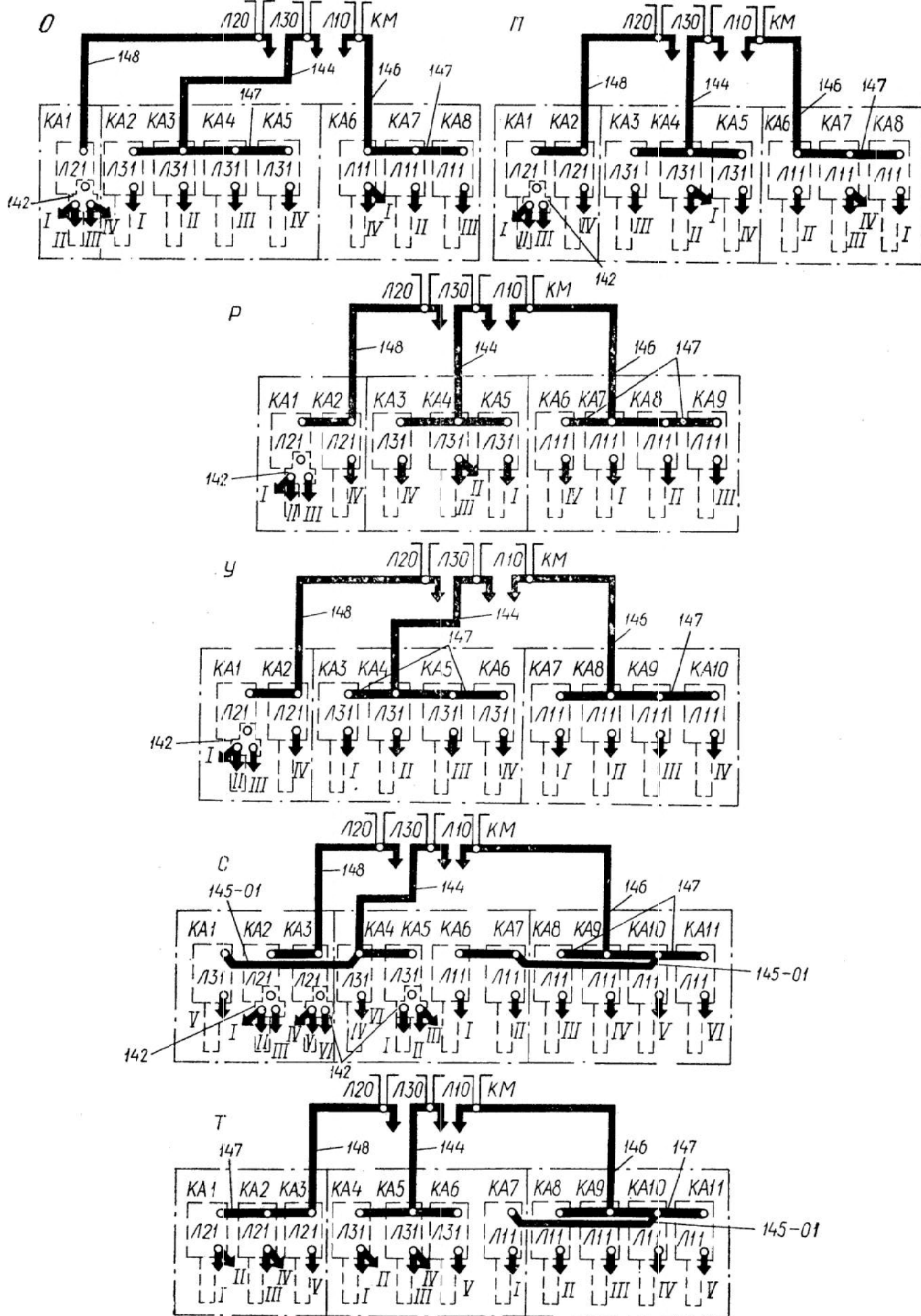
Схема электрическая соединений электромагнитов реле РЭО-401 для защитных панелей ПЗКБ-400У2.
